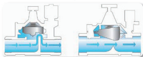
Labyrinthe droit sans déviation - Ultraflow
